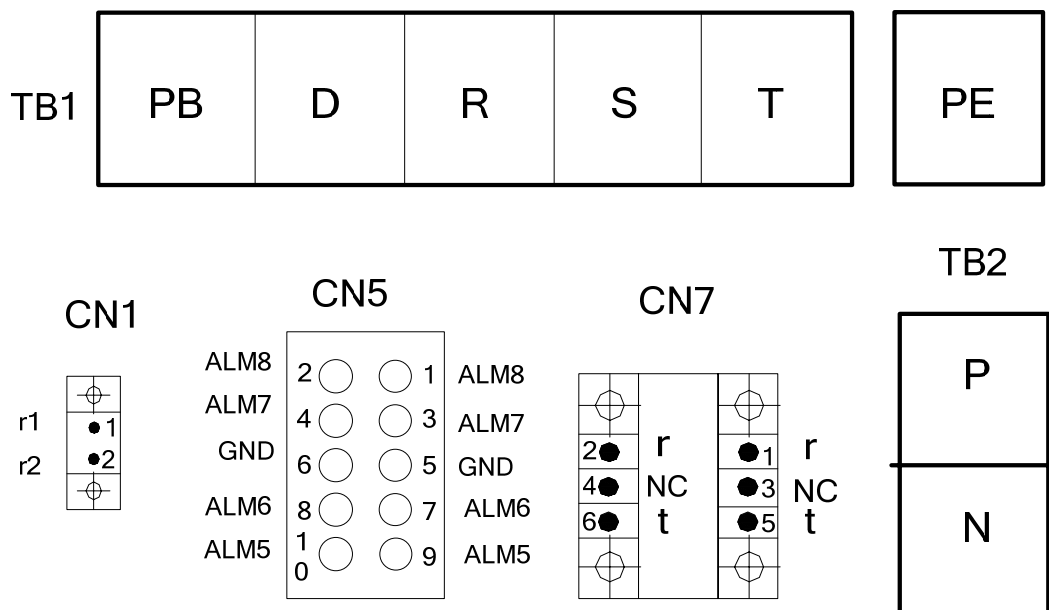
图 3-1 DTS02A-POW 端子图
