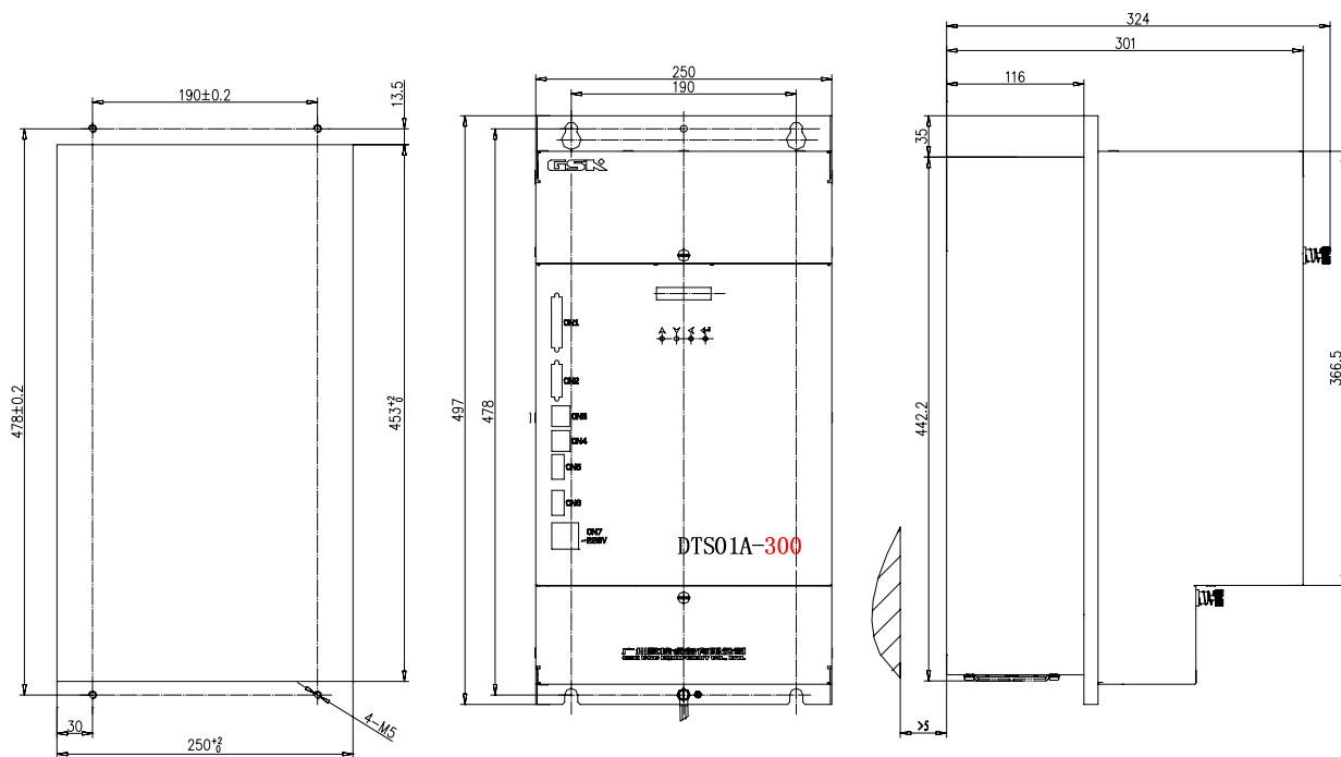
图 2-1 (d) DTS01A-300 开口尺寸图
