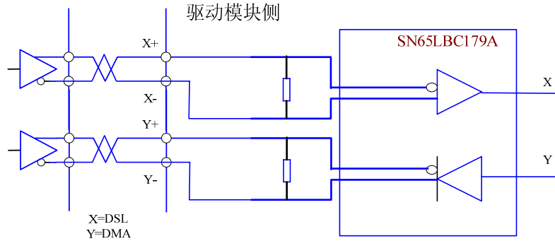
图 3-11 绝对式光电编码器输入接口
