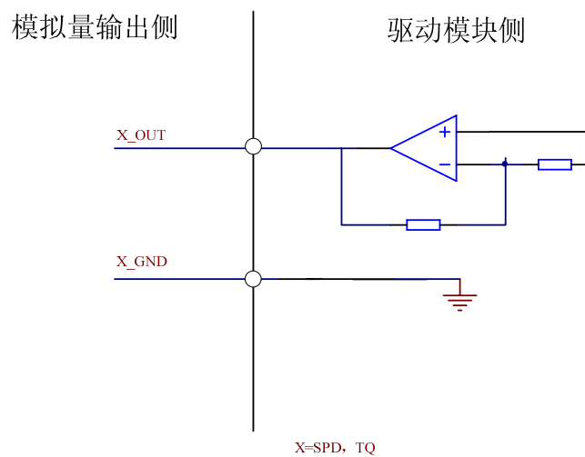
图 3-10 模拟量输出电路
