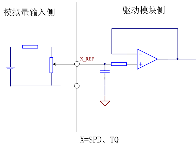
图 3-9 模拟量输入电路
