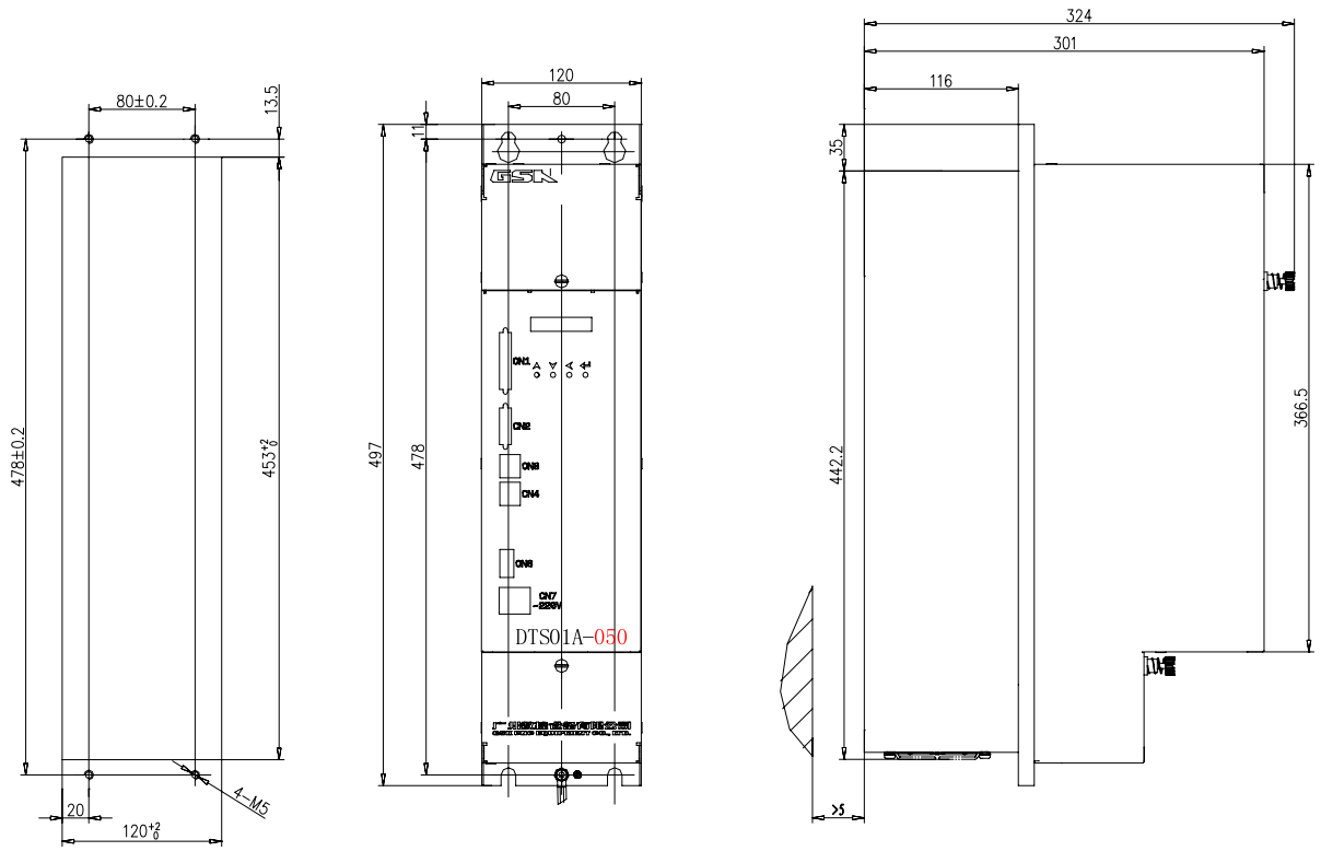
图 2-1 (b) DTS01A-050 开口尺寸图
