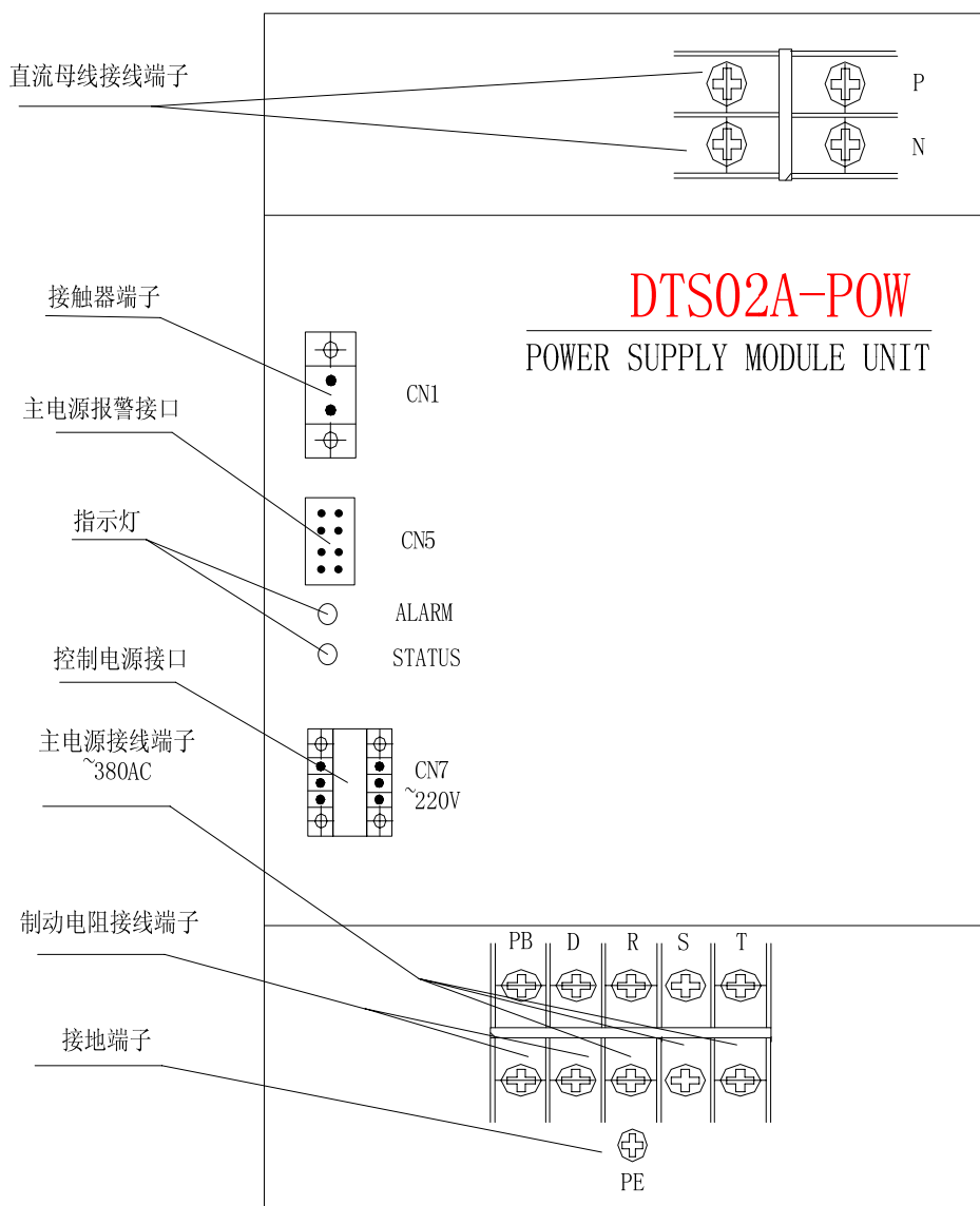
图 1-1 AE50 全电动注塑机专用驱动单元电源模块外观图
