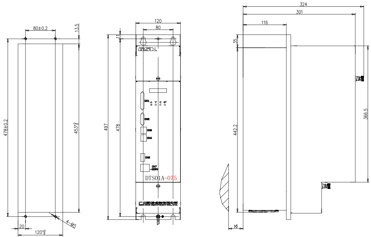
图 2-1 (c) DTS01A-075 开口尺寸图
